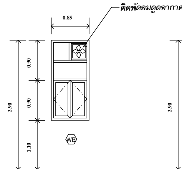
หน้าต่างบานเปิดคู่ วงกบ เหล็ก พ่น อบสี เทาเข้ม บานเปิด กรอบบานเหล็ก กระดาษ 6 มม. อุปกรณ์ บานเปิด มือจับ กุญแจล็อก ครบชุด
