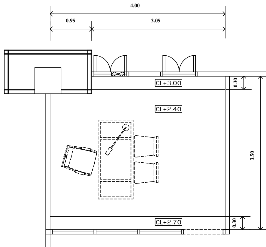
แปลนผ้าเพดานห้อง 102 Scale 1:50
