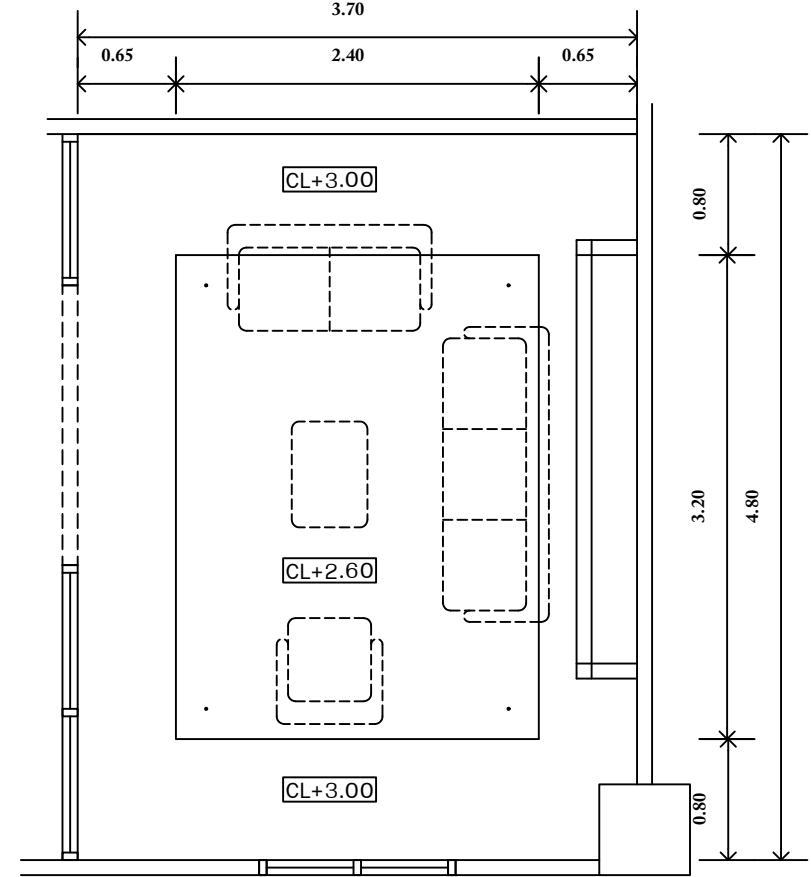
แปลนฝ้าเพดานห้อง 105 Scale 1:50
