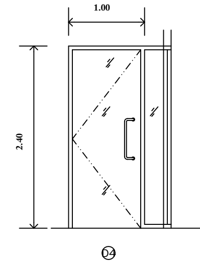
ประตูบานเปิดเดี่ยว วงกบ อลูมิเนียม เทาเข้ม บานเปิดกระดาษ 8 มม. เปลือย อุปกรณ์ บานเปิด กุญแจล็อก ครบชุด มือจับ สเตนเลส
