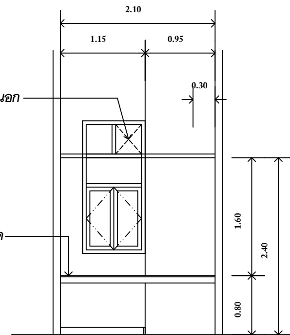
1 รูปด้านห้อง 106 Scale 1:50
