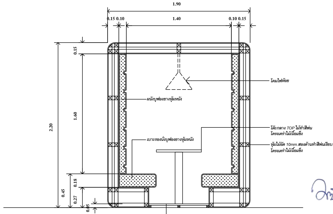
รูปตัด scale 1:25
