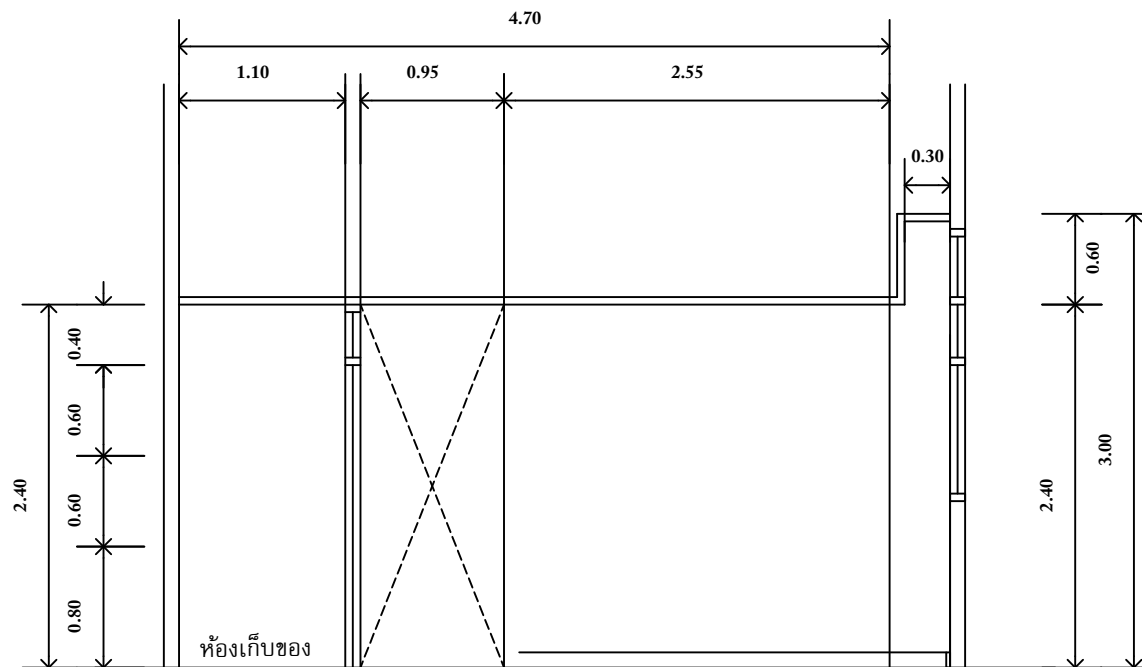
4 รูปด้านห้อง 106 Scale 1:50
