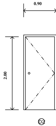
ประตูบานเปิดเดี่ยว วงกบ อลูมิเนียม เทาเข้ม บานเปิดไม้อัดท่อน้ำ กรู LAMINATED อุปกรณ์ บานเปิด มือจับ กุญแจล็อก ครบชุด
