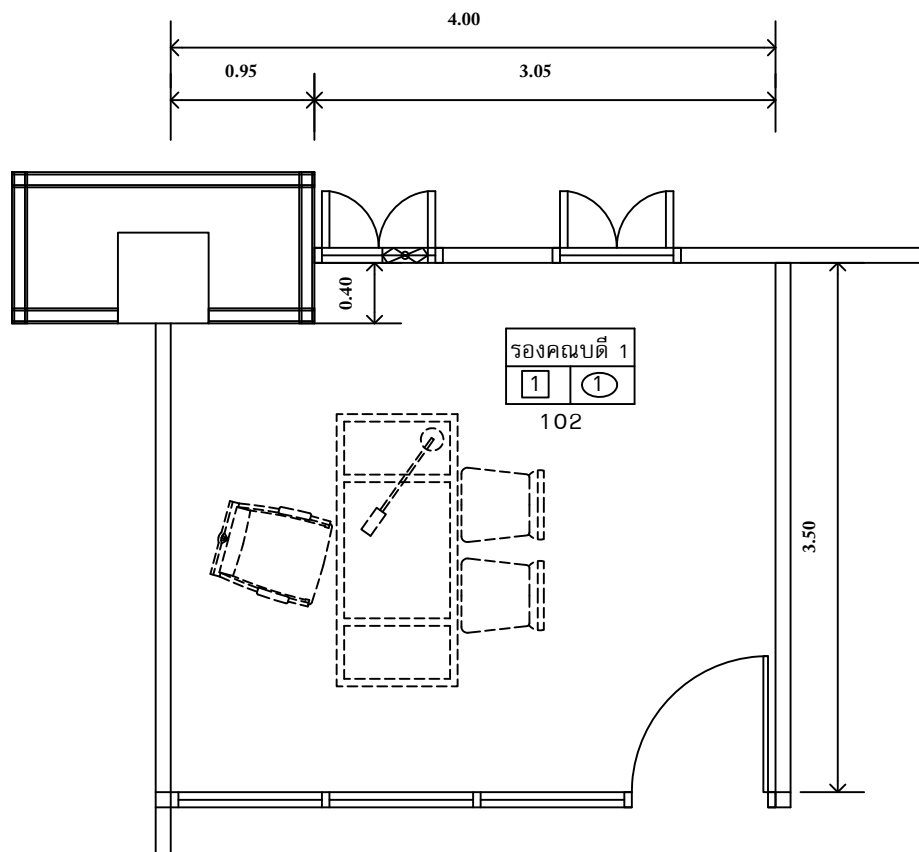
แปลนเฟอร์นิเจอร์ห้อง 102 Scale 1:50
