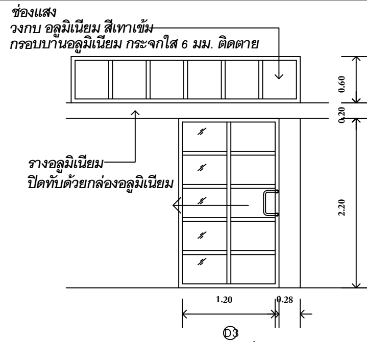
ประตูบานเลื่อน วงกบ อลูมิเนียม เทาเข้ม กรอบบานอลูมิเนียม กระดาษ 6 มม. อุปกรณ์รางเลื่อน กุญแจล็อก ครบชุด มือจับ สเตนเลส
