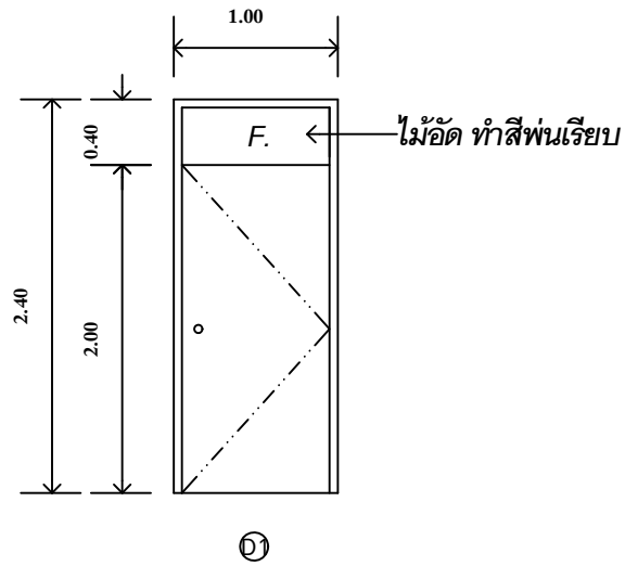
ประตูบานเปิดเดี่ยว วงกบ อลูมิเนียม เทาเข้ม บานเปิดไม้อัด ทำสีพ่นเรียบ อุปกรณ์ บานเปิด มือจับ กุญแจล็อก ครบชุด
