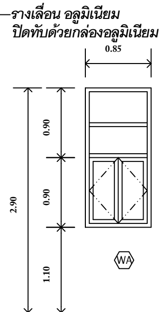
หน้าต่างบานเปิดคู่ วงกบ เหล็ก พ่น อบสี เทาเข้ม บานเปิด กรอบบานเหล็ก กระดาษ 6 มม. อุปกรณ์ บานเปิด มือจับ กุญแจล็อก ครบชุด
