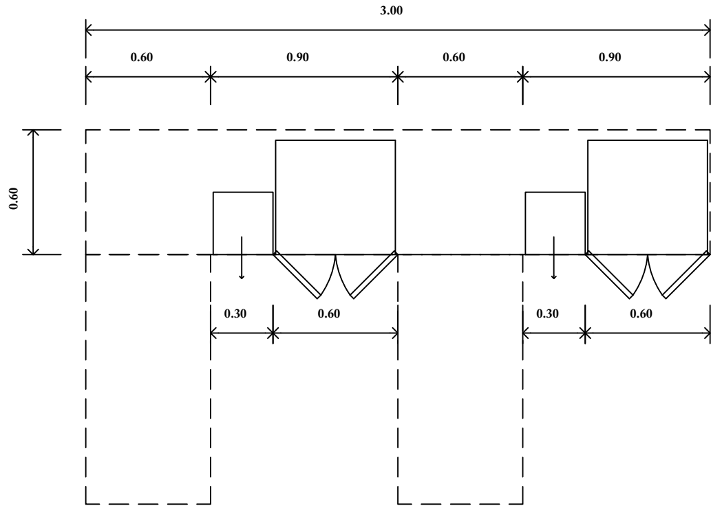
แปลนขยาย B110-3 scale 1:25
